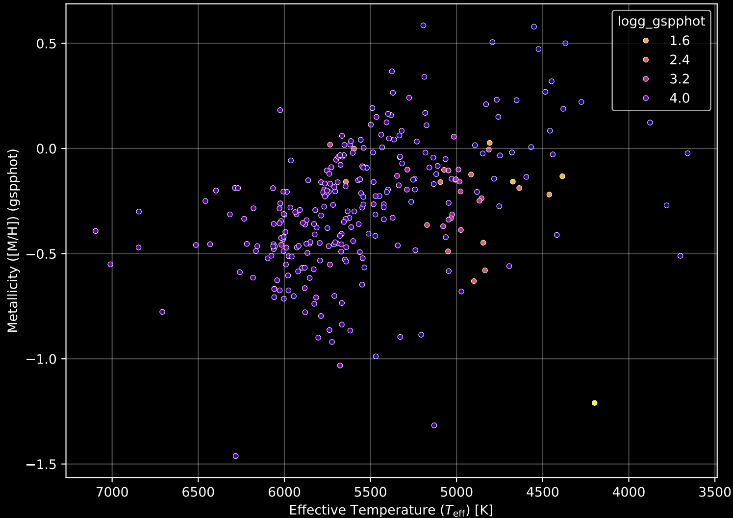
GALAH DR4 Field: [7008] Stellar Population Parameters (n= 288)
