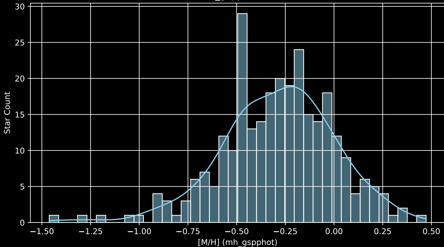
GALAH DR4 Field: [7008] [M/H] (mh_gspphot) (n= 284)
